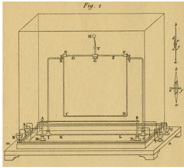
Når man sender en strøm gennem de to ledere i dette apparat, vil den ene bevæge sig. Fra Ampères Recueil d'observations électrodynamiques , 1822. Foto: Teknologihistorie DTU
