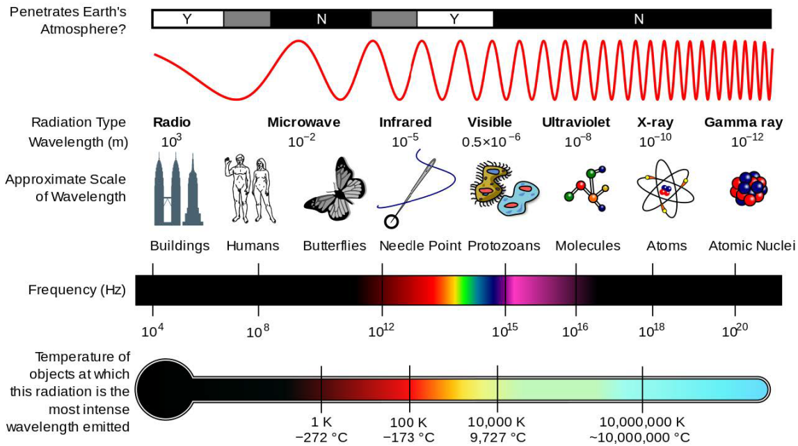
Det elektromagnetiske spektrum. Foto: Inductiveload, NASA - self-made, information by NASA https://commons.wikimedia.org/w/index.php?curid=2974242
