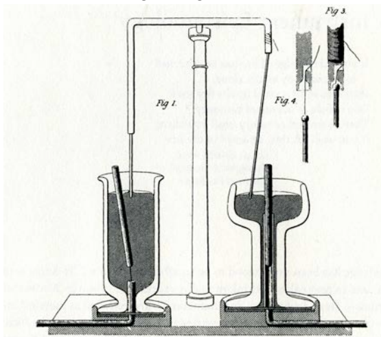
Faradays apparat, hvor en strømførende ledning roterede om en magnet og omvendt. Fra Experimental Researches in Electricity 1844. Foto: Wikicommons
